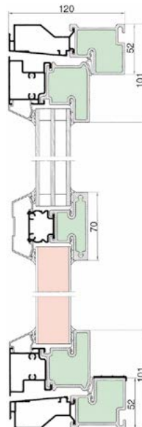
Fönsterdörr
