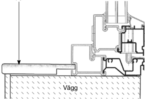
Ritning för infästning av smyg i våra fönster
