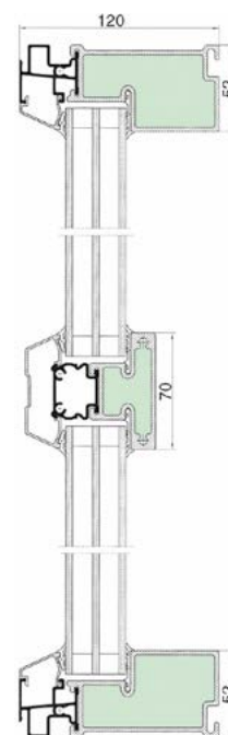
Fast fönster
