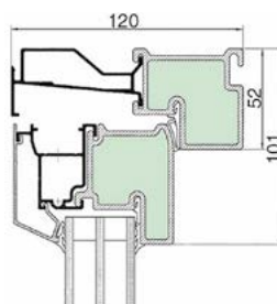
Detalj öppningsbart fönster
