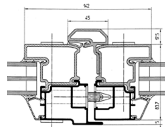
Pardörr 3-glas, mittanslag
