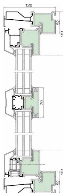
Öppningsbart fönster
